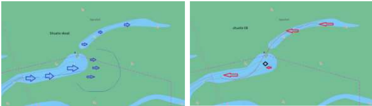
Fig.4 Stroomrichting bij vloed (links) en bij eb (rechts) op de voorkeurslocatie Sprutel, gelegen in een vloedsgaas
